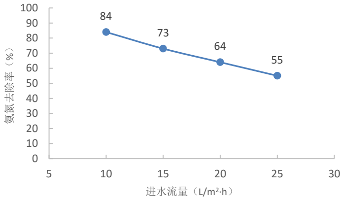
壳程进水流量与氨氮去除率关系曲线
