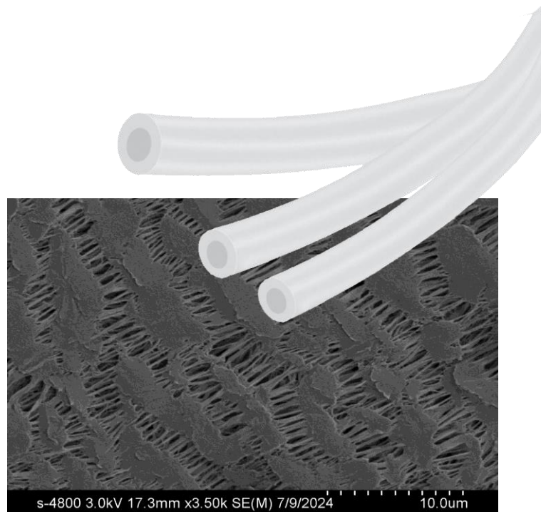
膜丝三维画图及 内表面3000倍电镜图
